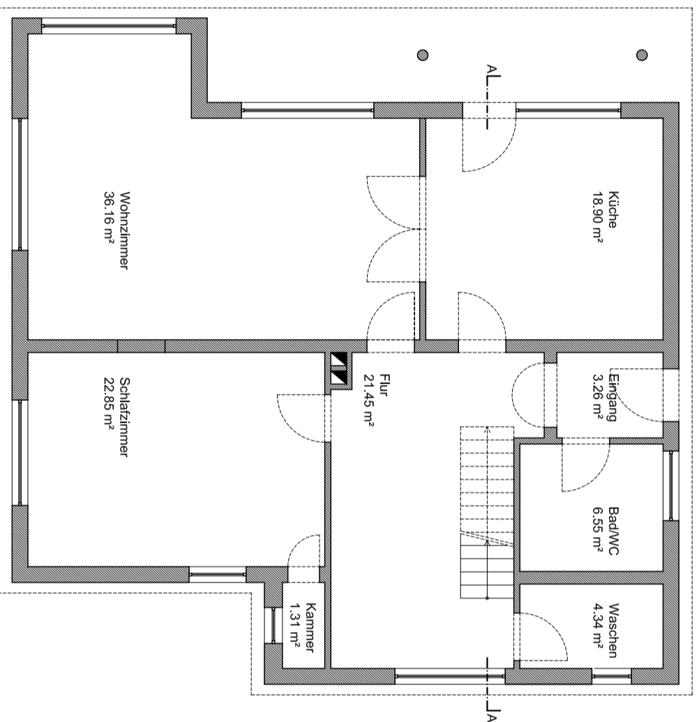
Grundriss Erdgeschoss Gesamt 114,82 m²
