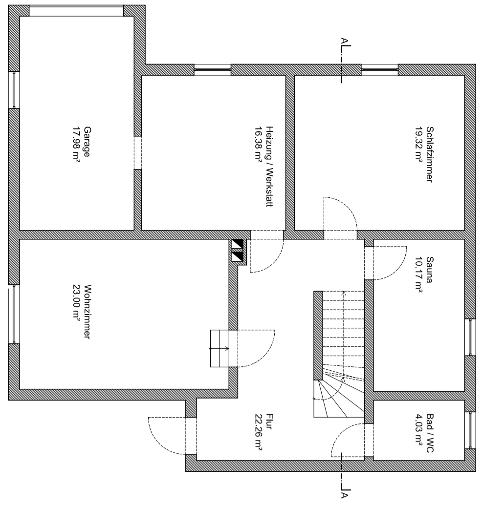
Grundriss Kellergeschoss Gesamt 113,14 m²
